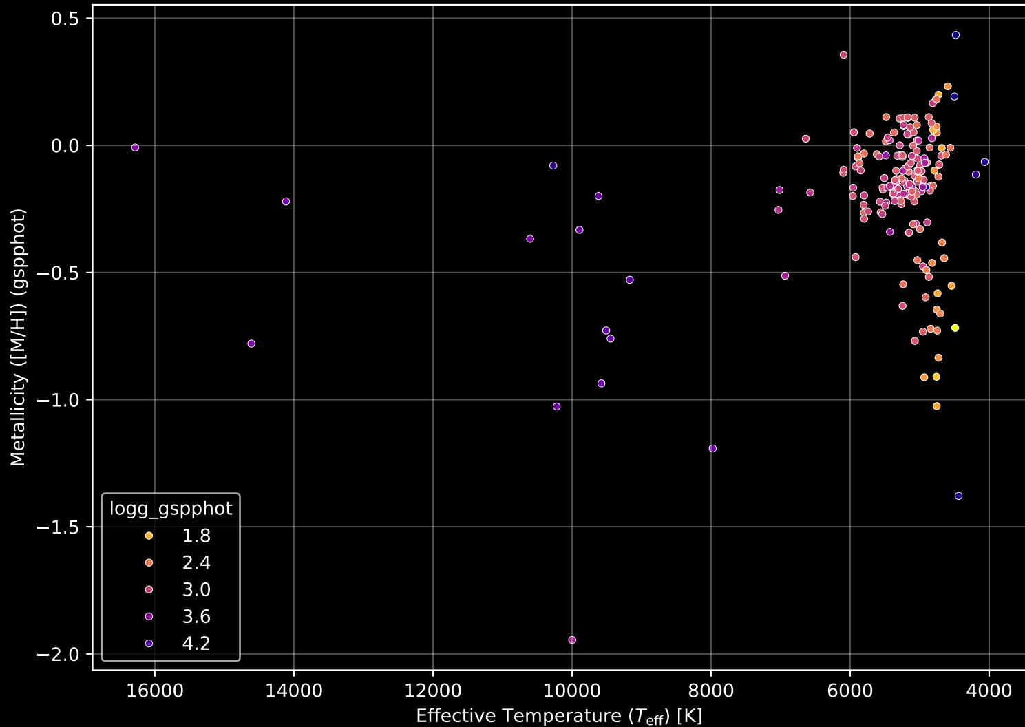
APOGEE DR17 Field: [161+04] Stellar Population Parameters (n= 193)
